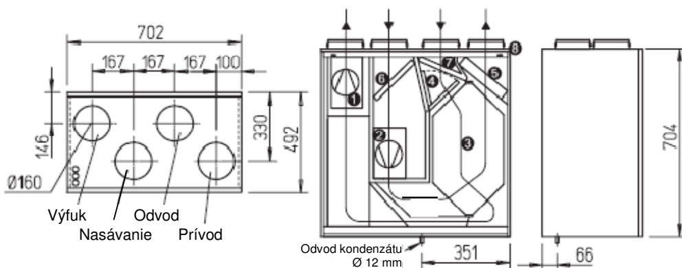
Obr. KWL EC 500 Pro L, vyhotovenie „ľavé“
