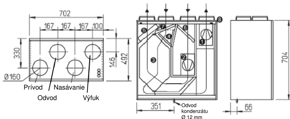
Obr. KWL EC 500 Pro R, vyhotovenie „pravé“
